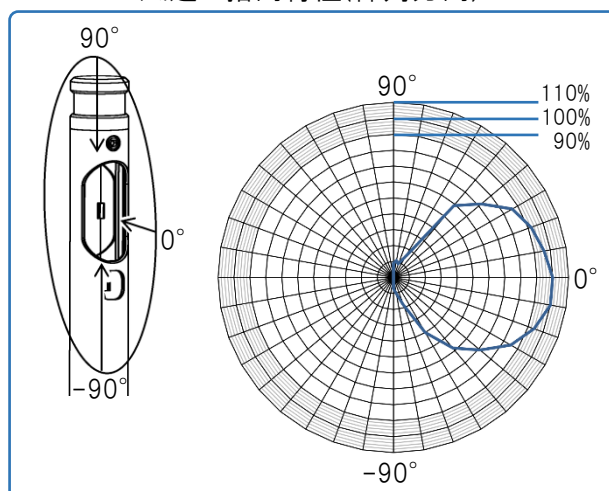
風速の指向特性(仰角方向)
