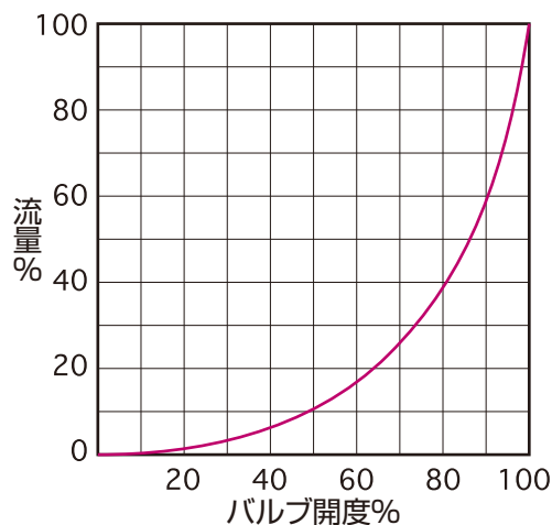
バルブ開度(%)に対する容量係数(Cv)
