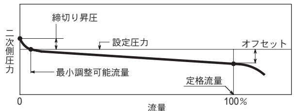
流量特性図
