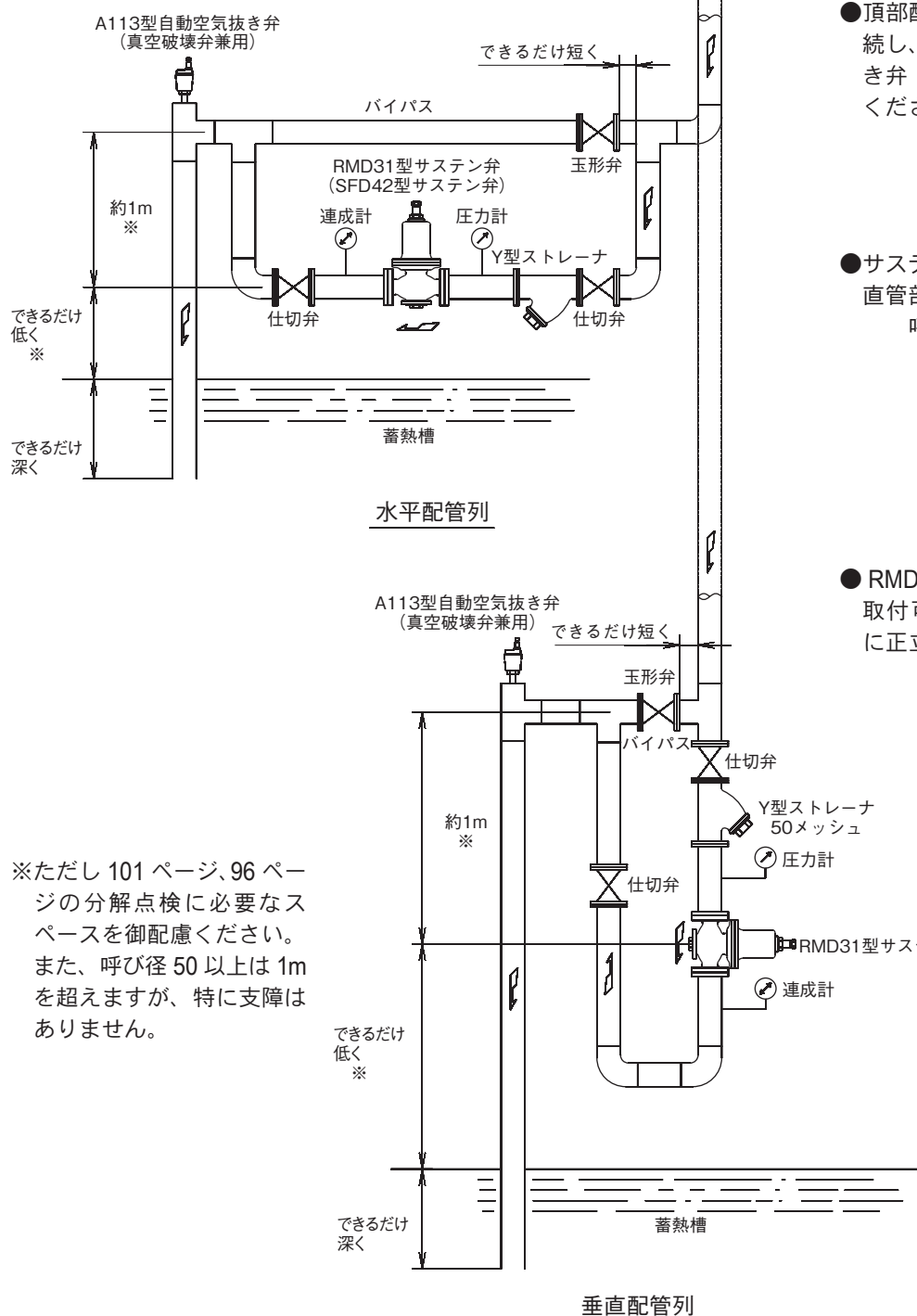
図11 配管例図
