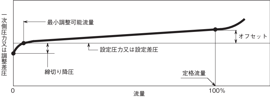
図4 サステン弁・差圧サステン弁 流量特性図
